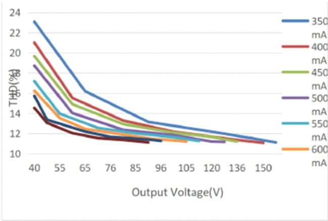
Зависимость полного гармонического искажения от выходного напряжения
