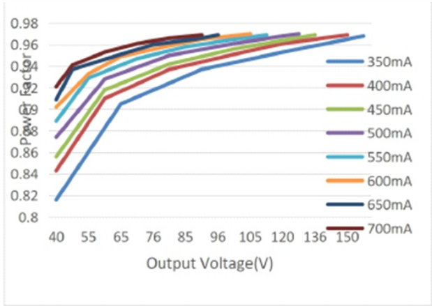
Зависимость коэффициента мощности от выходного напряжения
